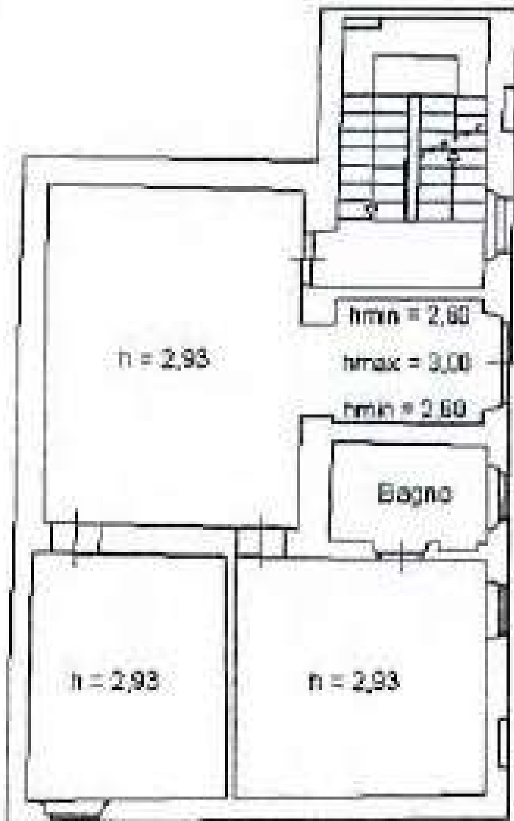
Piano Primo
